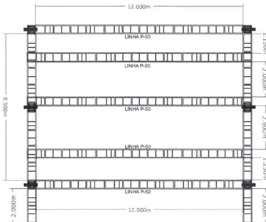
VISTA SUPERIOR
