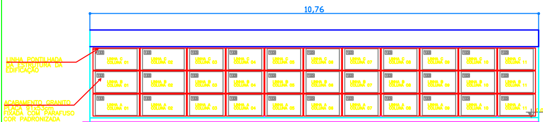
ELEV. 01 - COM TAMPA DE CONCRETO ESCALA.....1:50
