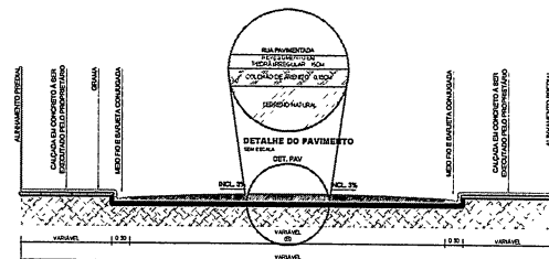
DET. SECÇÃO TRANSVERSAL DO PAVIMENTO
