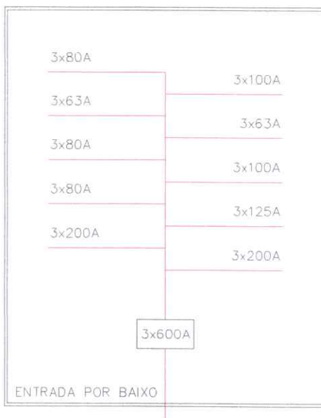
QUADRO DE DISTRIBUIÇÃO GERAL SEM ESCALA
