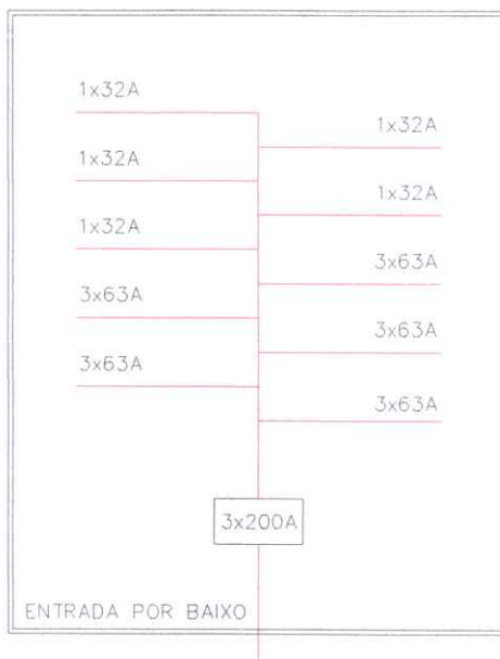
QUADRO DE COMANDO DO GERADOR SEM ESCALA
