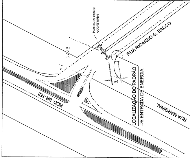
Detalhe Executivo Localização Padrão de Energia escala 1:1000
